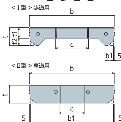
蓋寸法・重量< II型>
