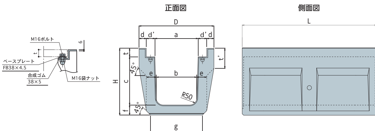
寸法表
