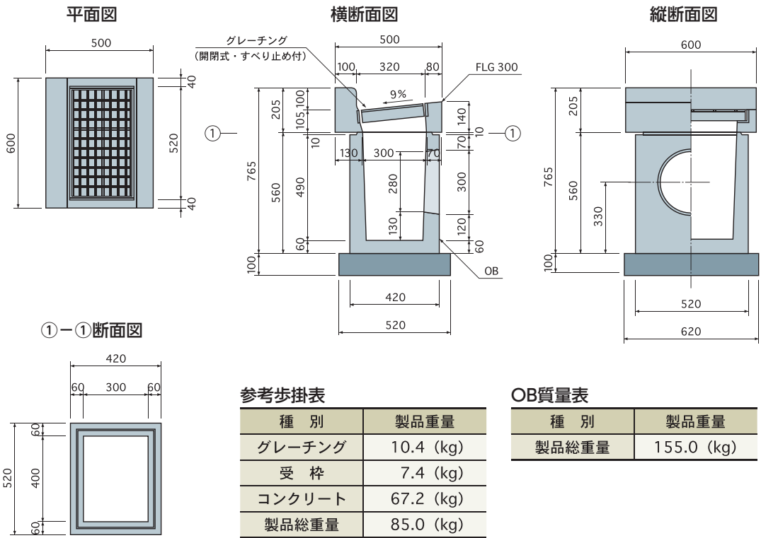
寸法図
