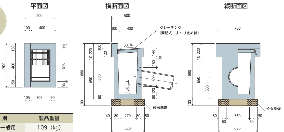
寸法図
