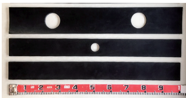
支承用ゴム クロロプレンゴム (CR) はHC床版と受台の間に使用します。
