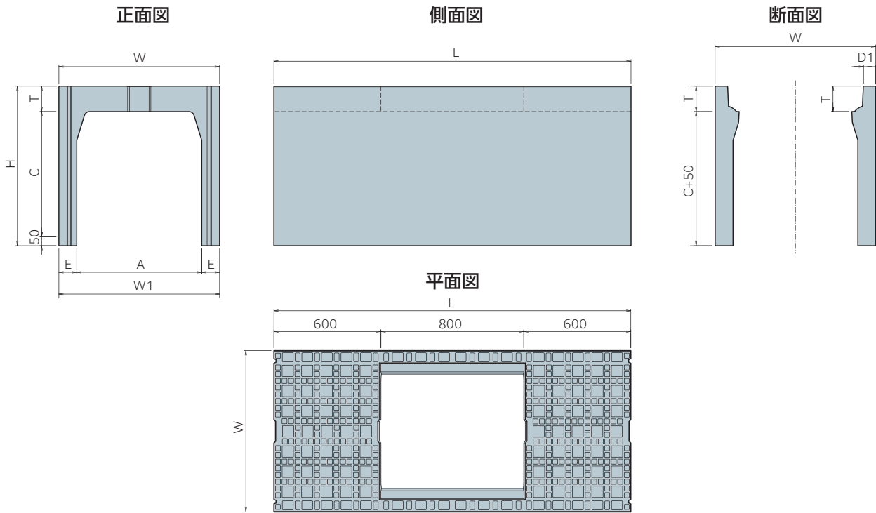
大型FX可変側溝 規格表 [700 シリーズ]
