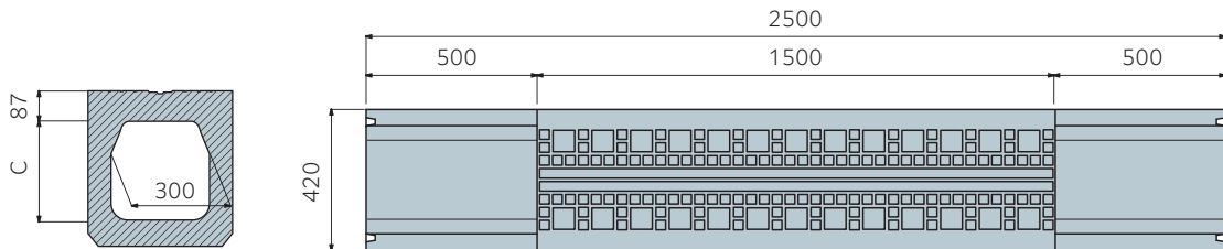
側溝平面図
