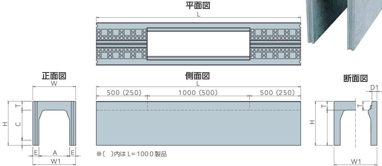
■ FX可変側溝(縦断用) 規格表 [250, 300 シリーズ]
