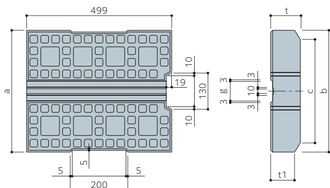
規格表 (車道用)
